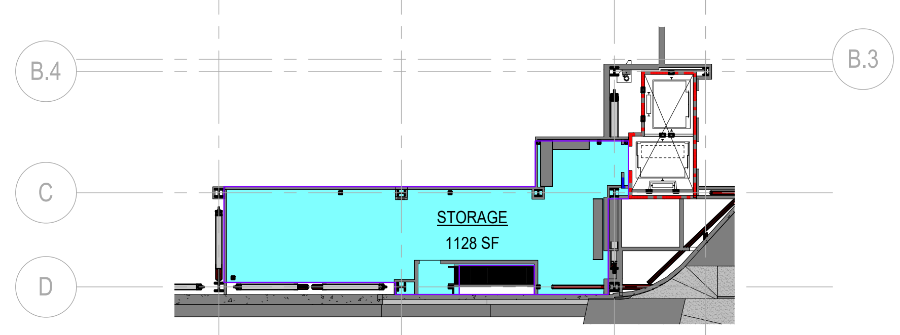
4 MEZZANINE LEVEL SCALE: 1/16" = 1'-0"
